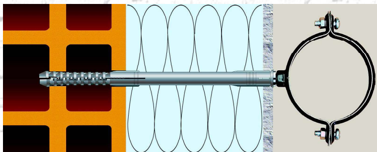
Rappresentazione montaggio Art. 316
